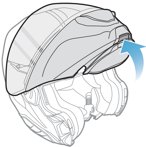
Casco modulare
